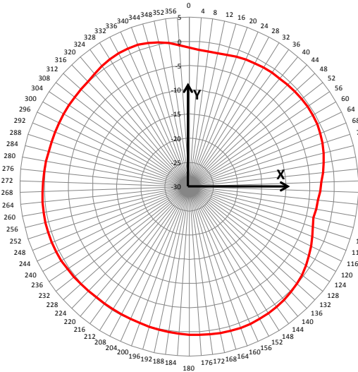
H-Plane
